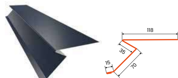
laštakis-karnizas mažas PHR
