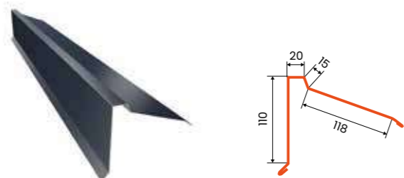
kraigas vienšlaičiam stogui PHR
