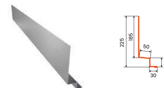
šoninis jungimas prie sienos PHR
